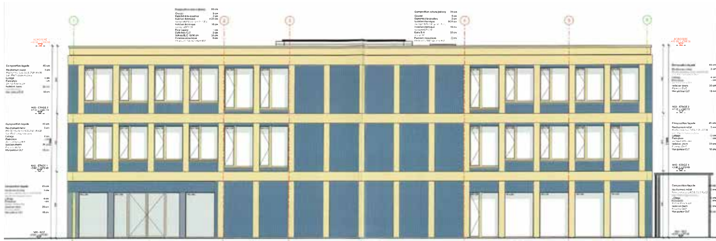
■ Plan de façade du collège CTR Arvel.
